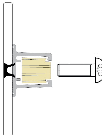
Vue en coupe Assemblage du rail
